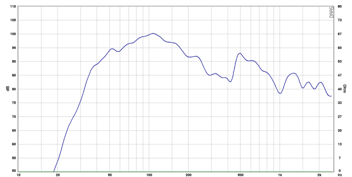
A8 Sub passiv Frequenzgangkurve
