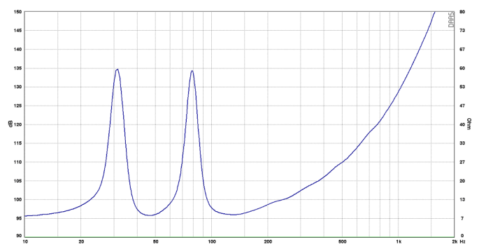
A8 Sub passiv Impedanzkurve
