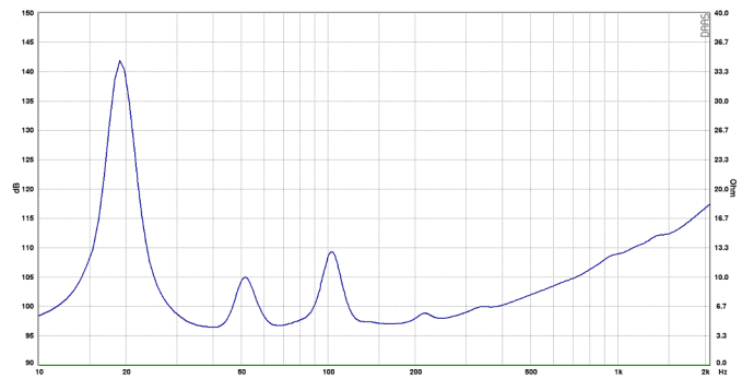
TSE infra Impedanzkurve
