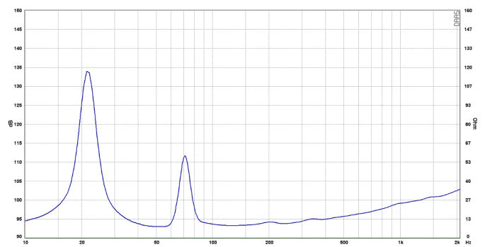
TSE Sub Impedanzkurve
